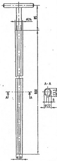
Σχήμα 5: Δειγματοληψτής τύπου Α
