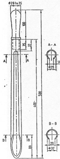
Σχήμα 6: Δειγματοληψτής τύπου Β
